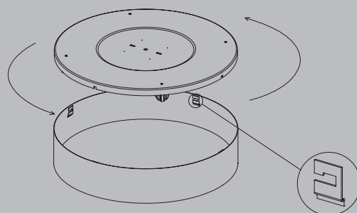
Trava de encaixe
